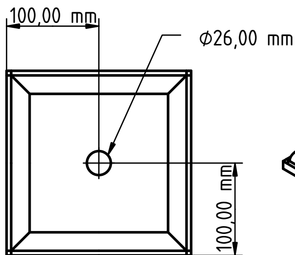
Draufsicht
