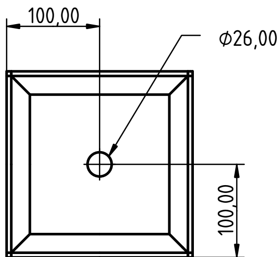
Draufsicht
